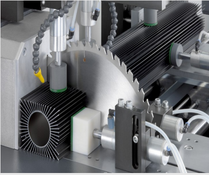
自动锯切机SAS 142/43
