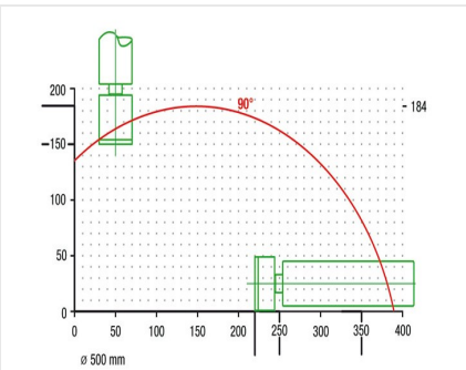
自动锯切机SAS 142/43
