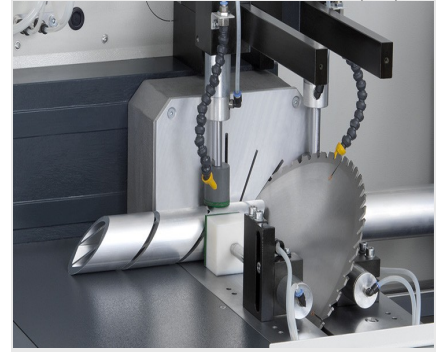
自动锯切机SAS 142/43
