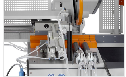
自动锯切机SA 73/36
