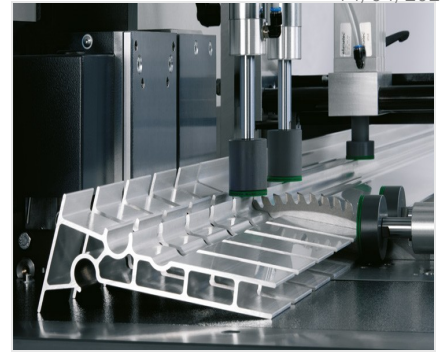
自动锯切机SA 142/38
