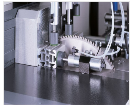
自动锯切机SA 142/37
