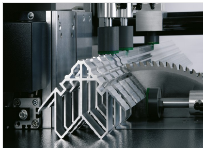
自动锯切机SA 142/38
