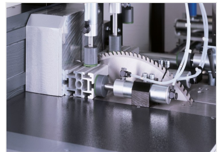
自动锯切机SA 142/37
