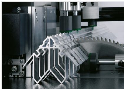
自动锯切机SA 142/38
