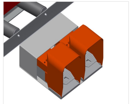
脚踏开关 通过脚踏阀门进行控制。在垂直位置上可以气动方式在500 mm的范围内调节高度，气动夹紧
