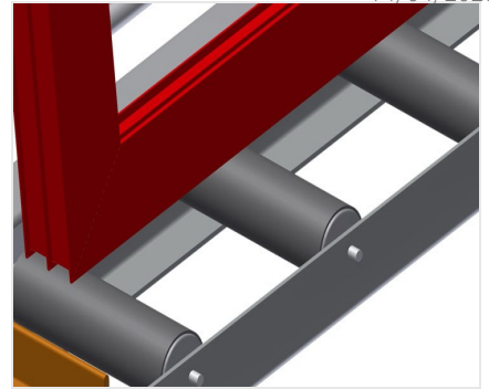
滚轮支承装置 带支承滚轮的下部滚道L = 200 mm
