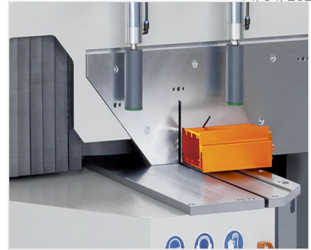
单头斜榫切割机MGS 105
