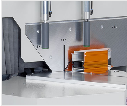
单头斜榫切割机MGS 105
