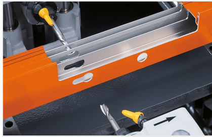
双轴仿形铣床KF 78/23
