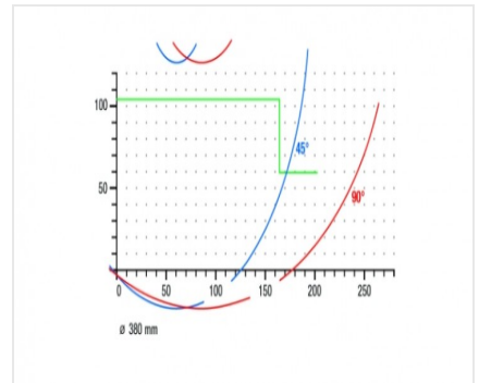
双头斜榫切割机DG 79 切割图DG 79
