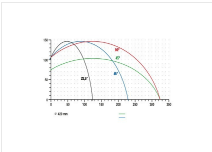
双头斜榫切割机DG 104 切割图DG 104
