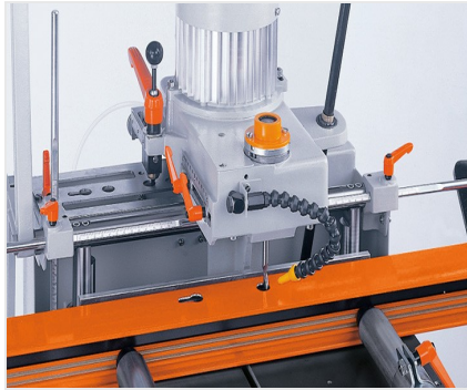
单轴仿形铣床AS 70/44
