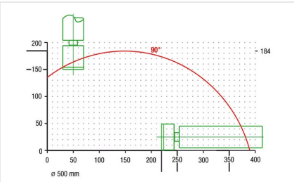
Otomatik Testere SAS 142/44
