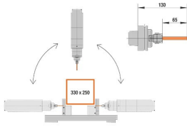
SBZ 140 Profil İşleme Merkezi
