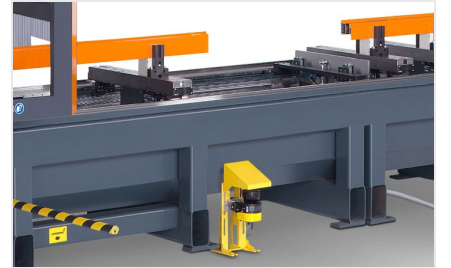
SBZ 140 Profil İşleme Merkezi
