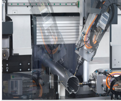
SBZ 140 Profil İşleme Merkezi
