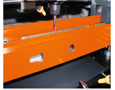
Üç Motorlu Kopya Freze KF 178/10
