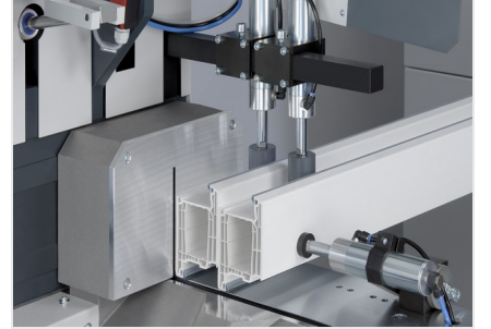
06. Çift Başlı Testere DG 142 XL
