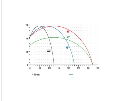
Çift Başlı Testere DG 104 Kesme Diyagramı DG 104
