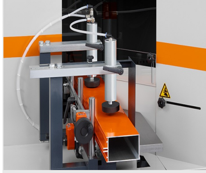
Profil Alıştırma Makinesi AKS V-550
