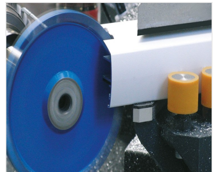
Обработка центр SBZ 631
