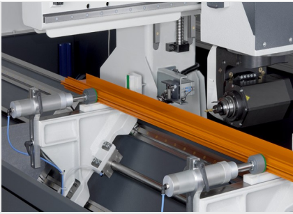
Обработывающий центр SBZ 122/74
