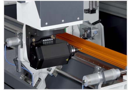
Регулировка угла с помощью оси A
