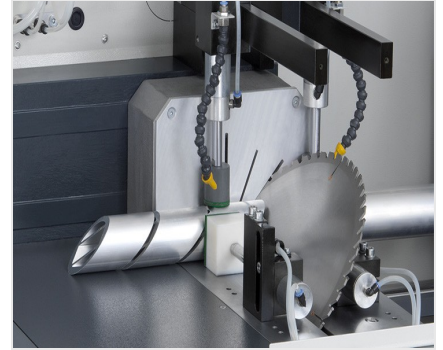
Пильный автомат SAS 142/43
