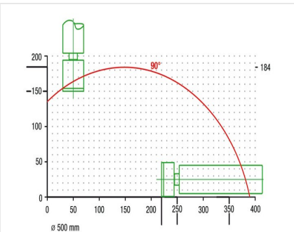
Пильный автомат SAS 142/43
