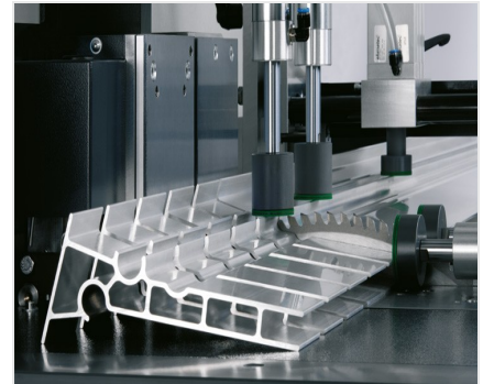
Пильный автомат SA 142/38
