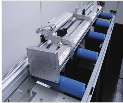
Упорно-измерительная система MMS 200
