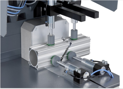
Ускоренная пила MGS 142/11
