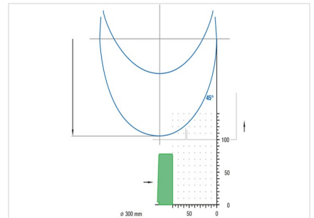
Пила для клиновых и торцевых вырезов KS 101/30
