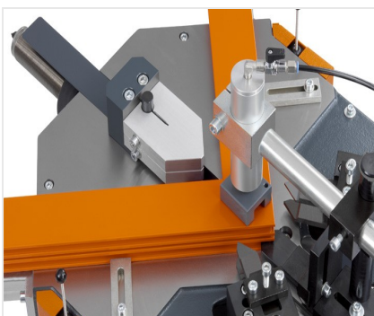
Пресс для стыковки углов EP 120
