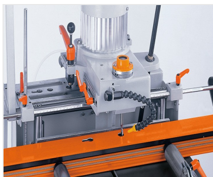
Одношпindelный копировально- фрезерный станок AS 70/44
