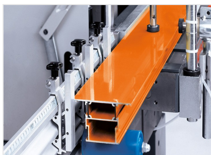
Одношпindelный копировально- фрезерный станок AS 170/10
