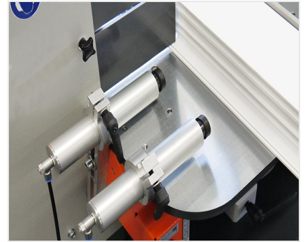
Фрезерный станок для фрезерования торцов AF 222/02
