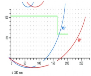
Máquina de corte angular MGS 73/33
