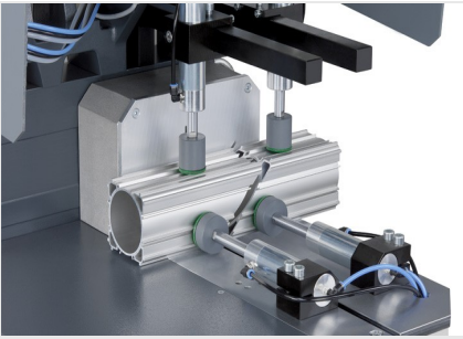
Máquina de corte angular MGS 142/11
