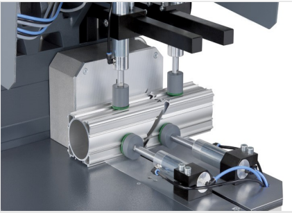
Máquina de corte angular MGS 142/11
