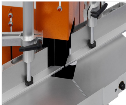
Máquina de corte em V KS 101/30
