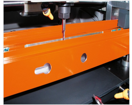
Fresa-copiadora de 2 cabeças KF 78/23
