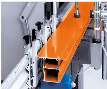
Fresa-copiadora de 1 cabeça AS 170/10
