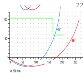
Piła obrotowa MGS 73/33
