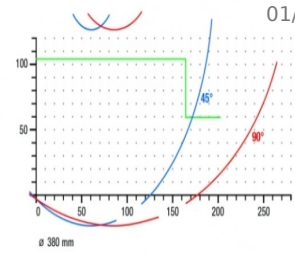
Piła obrotowa MGS 73/33
