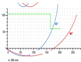
Piła obrotowa MGS 72/30 Diagram cięcia MGS 72/30
