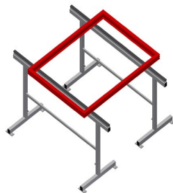
Stojaki montażowe (jedna para) MB 2000
