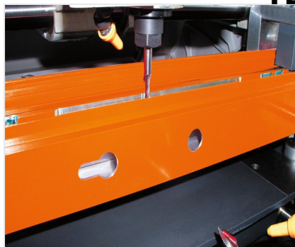
Dwuwrzcionowa frezarko-kopiarka KF 78/23
