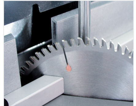
Tafelzaag TS 161/21
