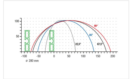
Tafelzaag TS 161
