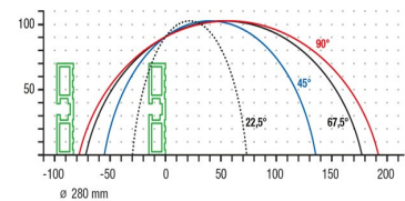
Tafelzaag TS 161
