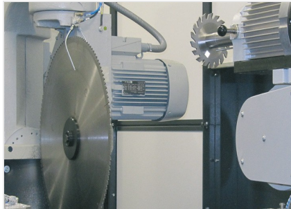
Profilbewerkingscentrum SBZ 631
