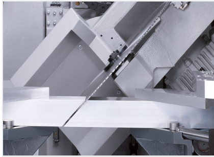
Profilbewerkingscentrum SBZ 631
