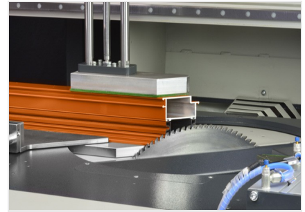
Zaagcentrum SBZ 616/02
