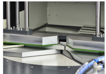
Zaagcentrum SBZ 616/02
