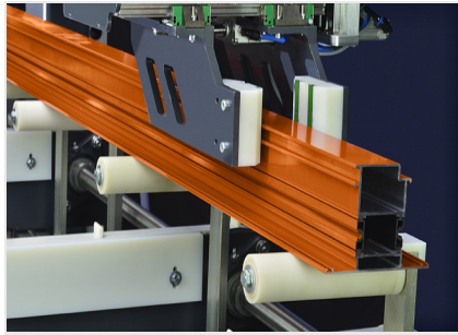
Zaagcentrum SBZ 616/02
