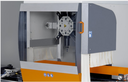
a- Profilbewerkingscentrum SBZ 131 eluCam
