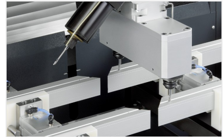
Profilbewerkingscentrum SBZ 131 eluCam
