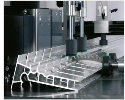
Zaagautomaat SAS 142/44
