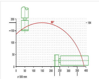
Zaagautomaat SAS 142/44
