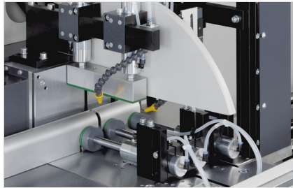
Zaagautomaat SAS 142/44
