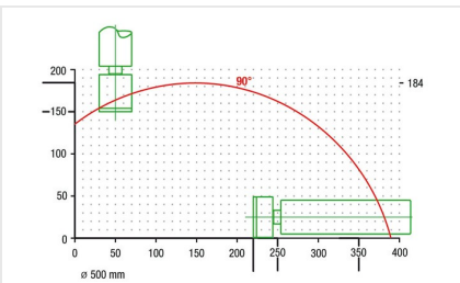
Zaagautomaat SAS 142/44
