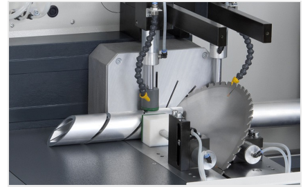
Zaagautomaat SAS 142/43
