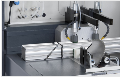
Zaagautomaat SAS 142/43
