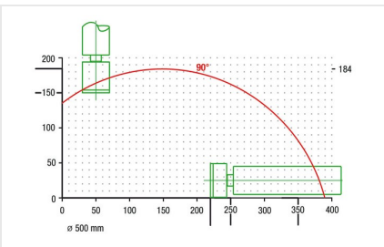
Zaagautomaat SAS 142/43
