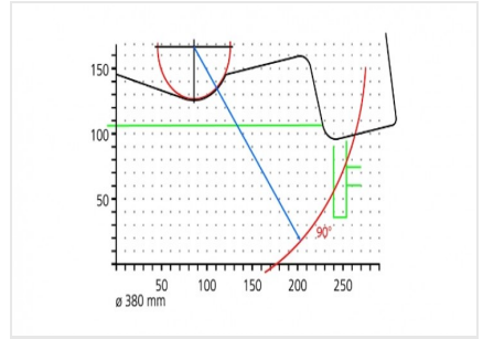
Zaagautomaat SA 73/36
