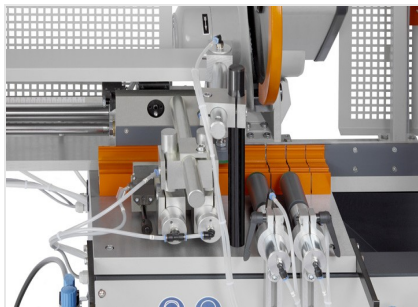
Zaagautomaat SA 73/36
