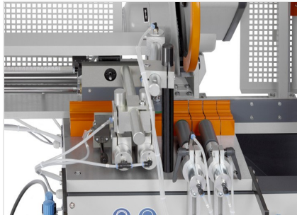
Zaagautomaat SA 73/36
