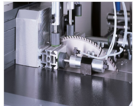
Zaagautomaat SA 142/37
