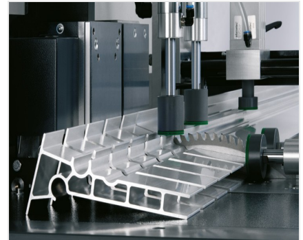
Zaagautomaat SA 142/38
