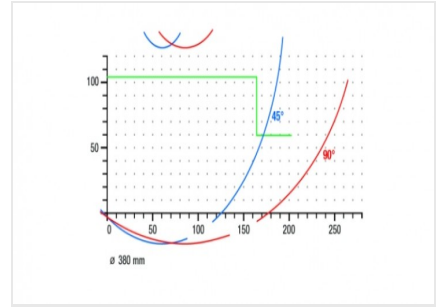
Verstekzaagmachine MGS 73/33
