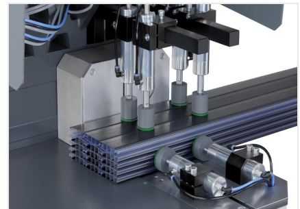
Verstekzaagmachine MGS 142/11
