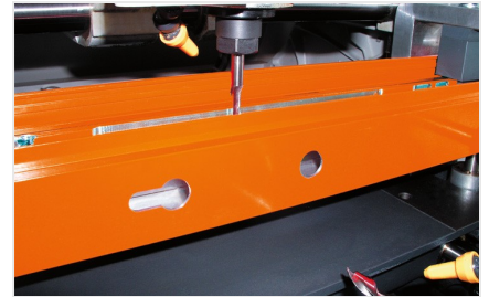
Tweespindel- kopieerfreesmachine KF 78/23
