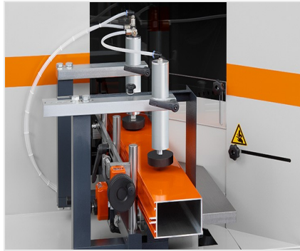
Uithoekzaagmachine AKS V-550
